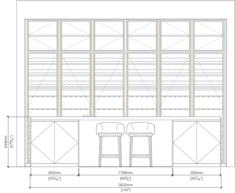
Elevation A
